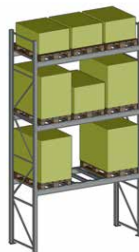
Abb. 4 Regal ohne SB-Integrierung lichte Feldweite \geq 2700 mm
