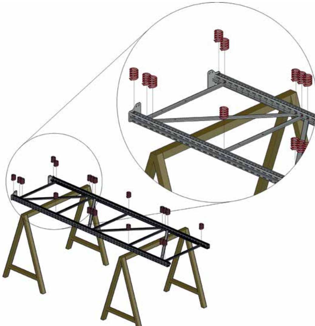
Abb. 56 Montage aller Füllstäbe – selbstfurchende Schrauben festziehen
