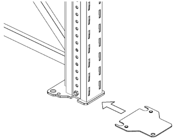
Abb. 75 Ausgleich von Bodenunebenheiten mittels Blechunterlage
