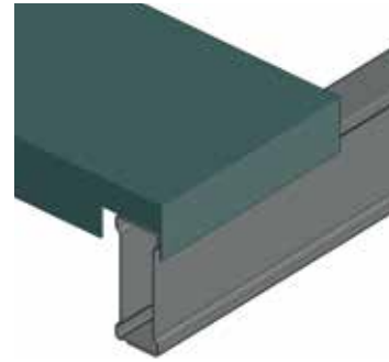
Abb. 35 ITD-Traverse mit aufgelegtem Einlegeboden
