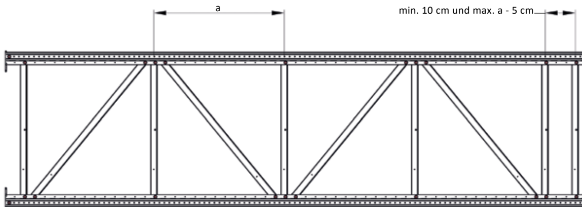
Abb. 58 Vollständig zusammengebauter Regalständer CG 55 x 40 mit zusätzlichem waagerechten Füllstab
