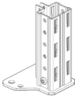
Abb. 12 Stützenprofil CG 55 x 40
