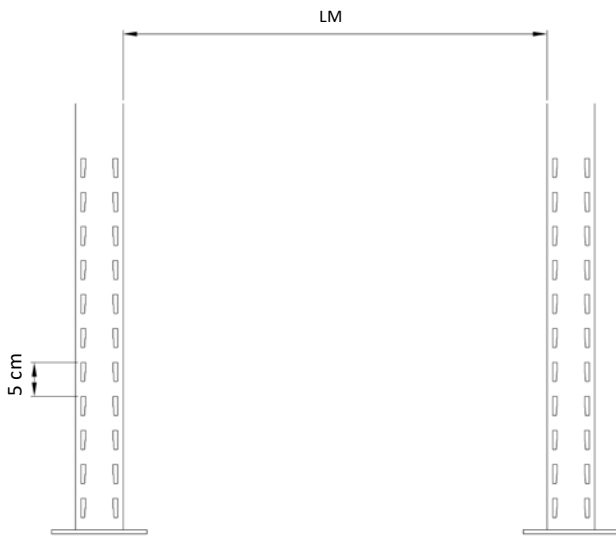
Abb. 26 Feldweite am System CI
