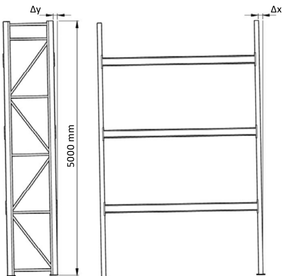
Abb. 87 Maximal zulässige Abweichung von der Lotrechten beim Betrieb von Regalen
