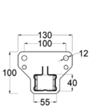
Abb. 17 Standard-Fußplatten der Stützenprofile (alle Maße in mm)
