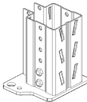
Abb. 15 Stützenprofil CI 85 x 80
