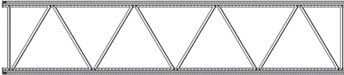
Abb. 67 Vollständig zusammengebauter Regalständer CI 100 x 80
