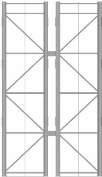
Abb. 40 Abstandshalter für System CG 50 x 40, CG 70 x 80 und CI 70 x 80
