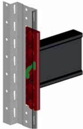
Abb. 21 Einsetzen der Aushebesicherung für das CG-System
