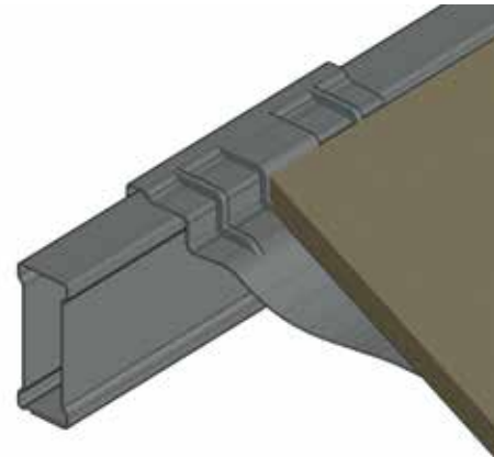
Abb. 34 Aufgelegte Spanplatte als Fachboden auf Tiefensteg FO abgesetzt
