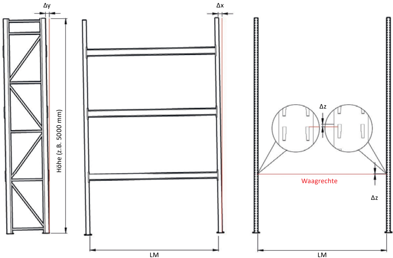
Abb. 74 Maximal zulässige Abweichung von der Lot- und Waagerechten bei der Montage von Regalen
