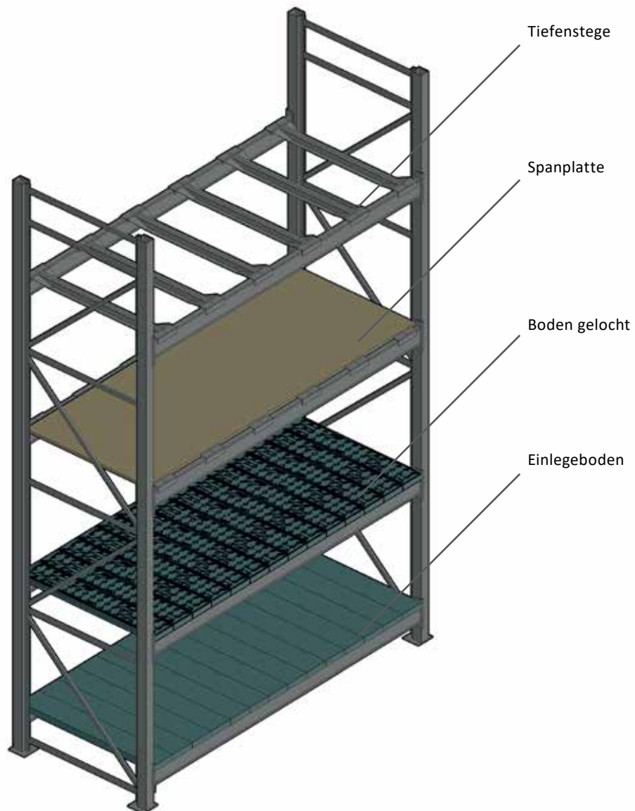
Abb. 39 Ein mit verschiedenen Böden bestücktes Schwerlastregal
