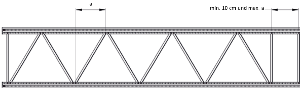
Abb. 68 Vollständig zusammengebauter Regalständer CI 100 x 80 mit zusätzlichem Füllstab
