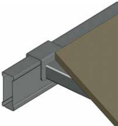
Abb. 33 Aufgelegte Spanplatte als Fachboden auf Tiefensteg abgesetzt
