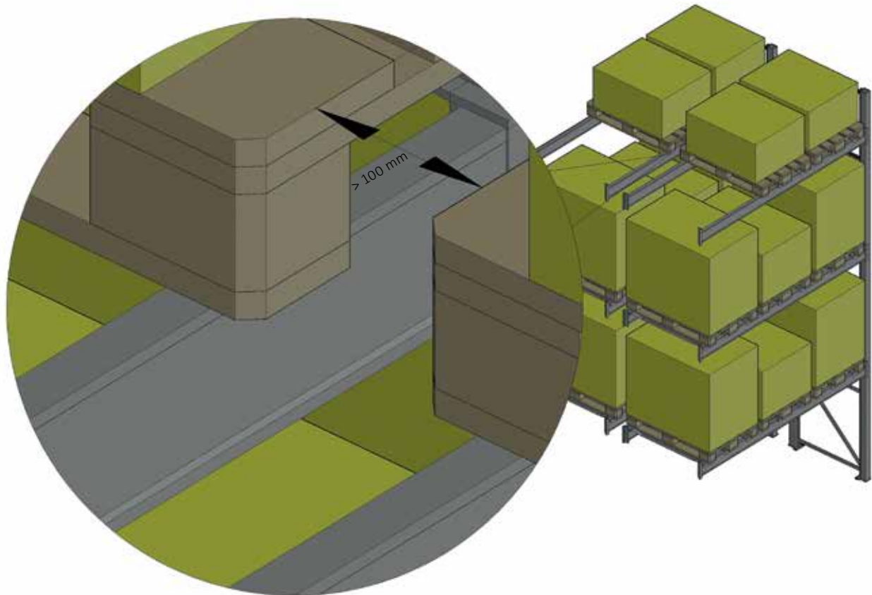
Abb. 6 Doppelregal ohne Durchschubsicherung
