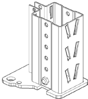
Abb. 14 Stützenprofil CI 70 x 80
