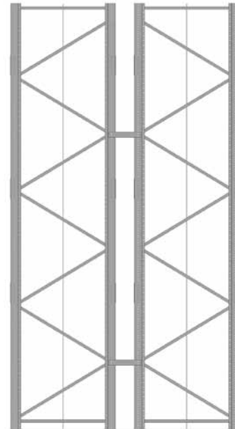
Abb. 42 Abstandshalter mit Füllstab- ausfachung im V-Muster
