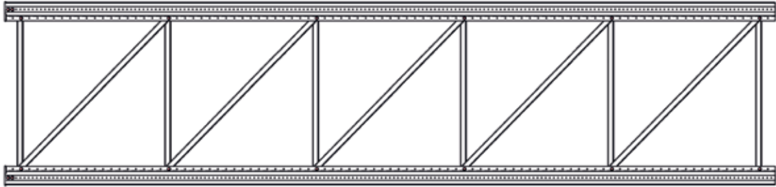
Abb. 73 Vollständig zusammengebauter Regalständer CI 100 x 80
