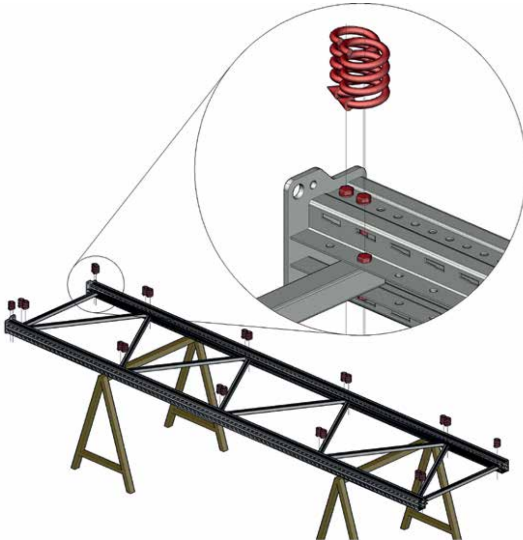
Abb. 66 Montage aller Füllstäbe – Schrauben festziehen
