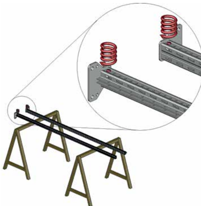
Abb. 49 Montage der Fußplatten mit selbstfurchenden Schrauben – Schrauben festdrehen
