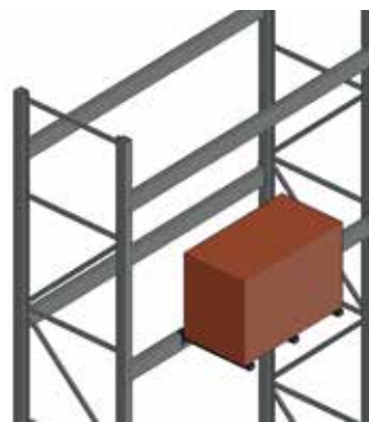
Abb. 80 Unzulässig auf Torsion belastete Traverse
