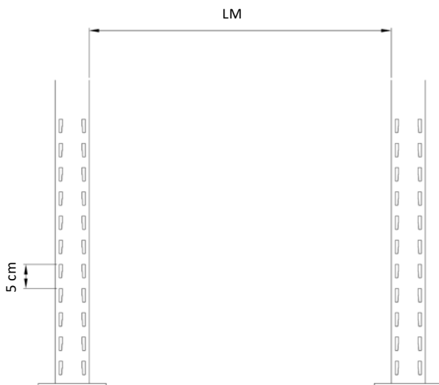
Abb. 25 Feldweite am System CG
