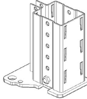
Abb. 13 Stützenprofil CG 70 x 80
