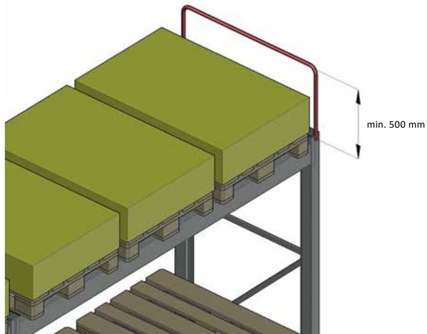
Abb. 8 Endständer mit Endbügel
