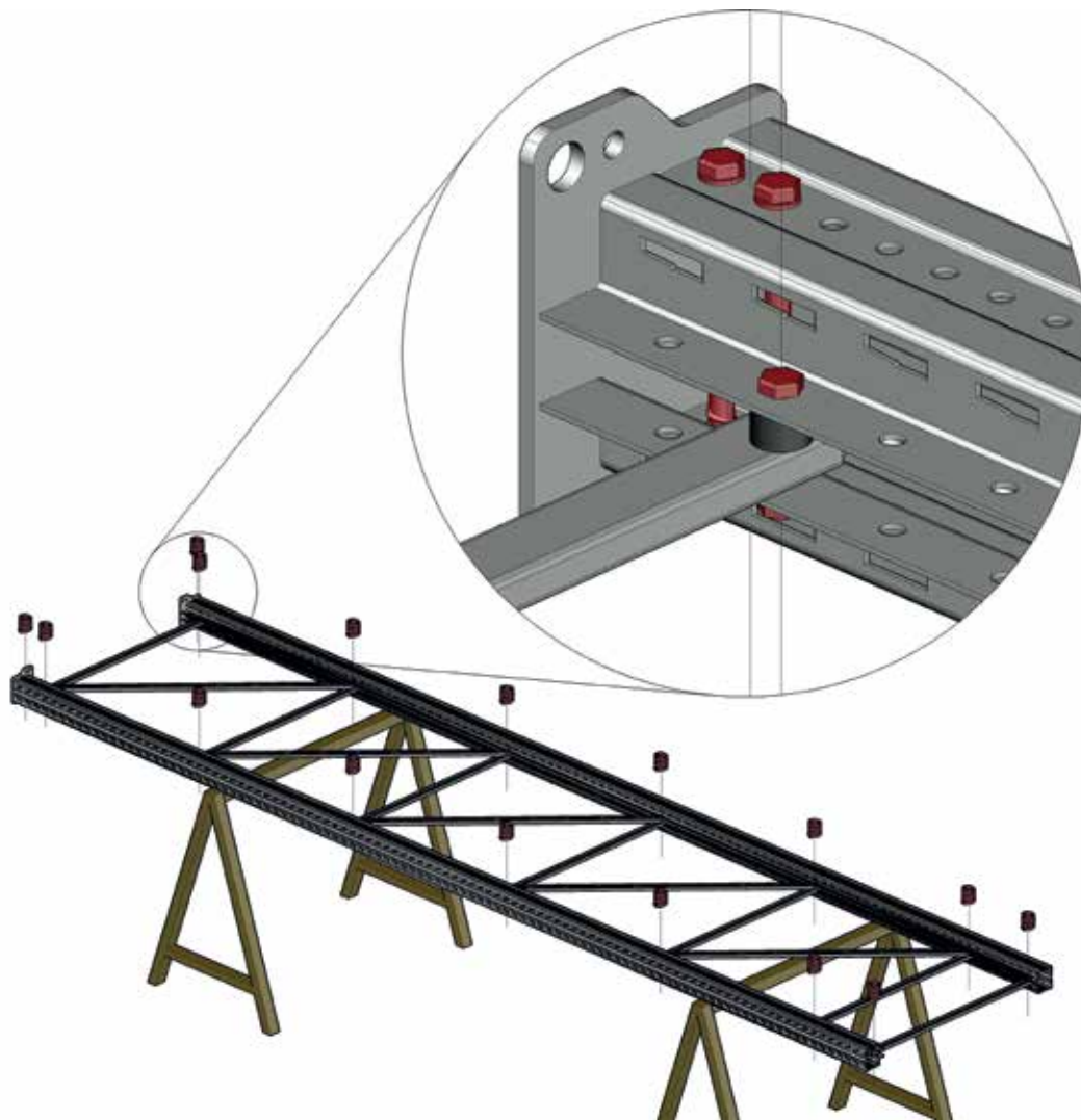
Abb. 71 Montage aller Füllstäbe – Schrauben festziehen
