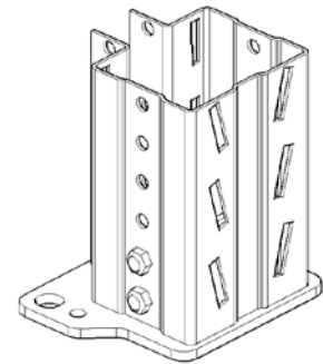
Abb. 16 Stützenprofil CI 100 x 80
