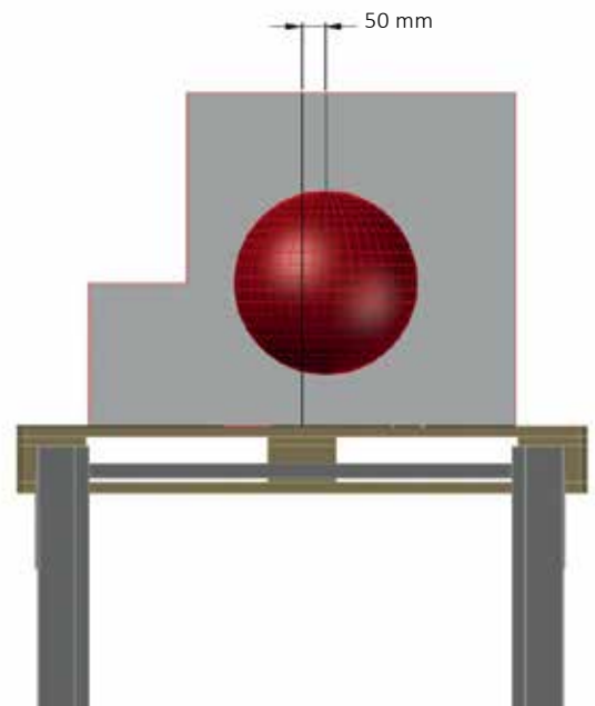
Abb. 10 Maximal zulässiger Versatz des Lastschwerpunktes zur Mittelachse
