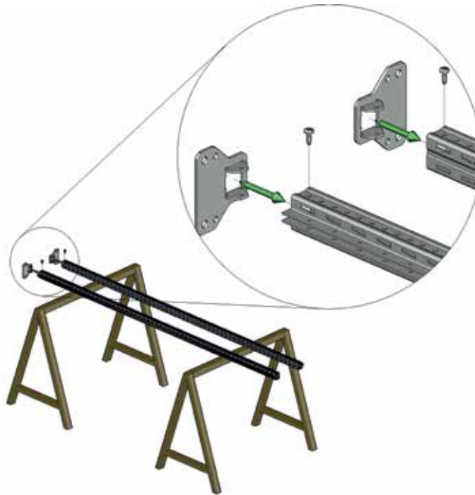
Abb. 48 Montage der Fußplatten mit selbstfurchenden Schrauben
