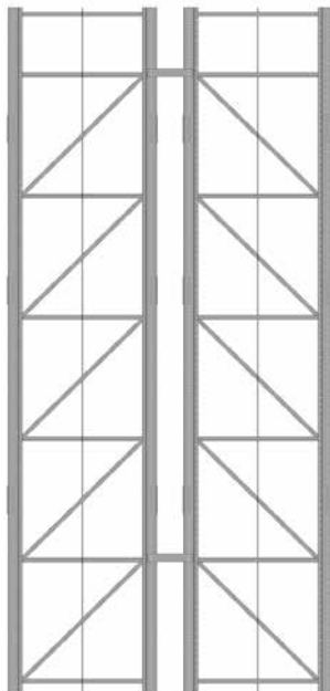
Abb. 41 Abstandshalter mit Füllstab- ausfachung im M-Muster
