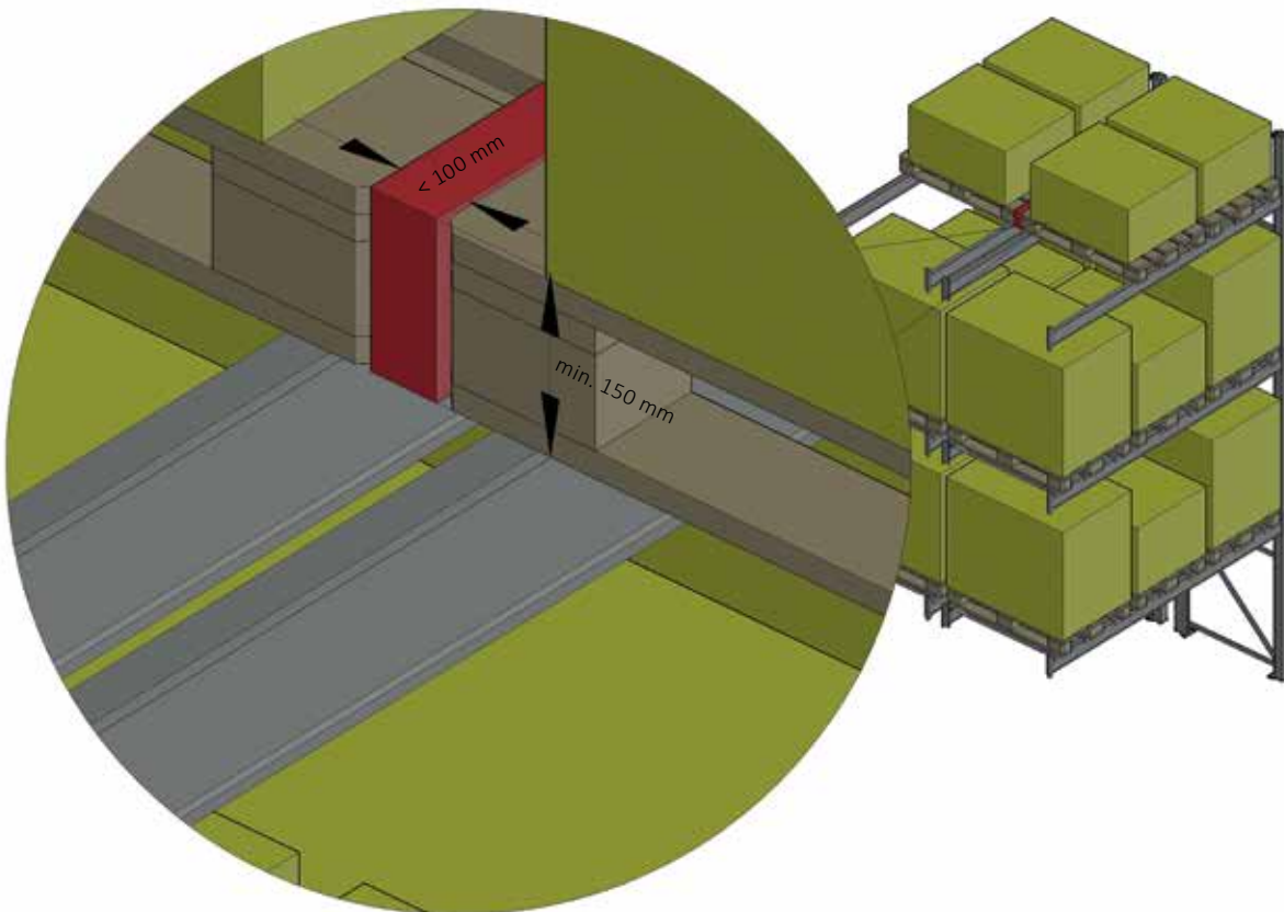
Abb. 5 Doppelregal mit Durchschubsicherung
