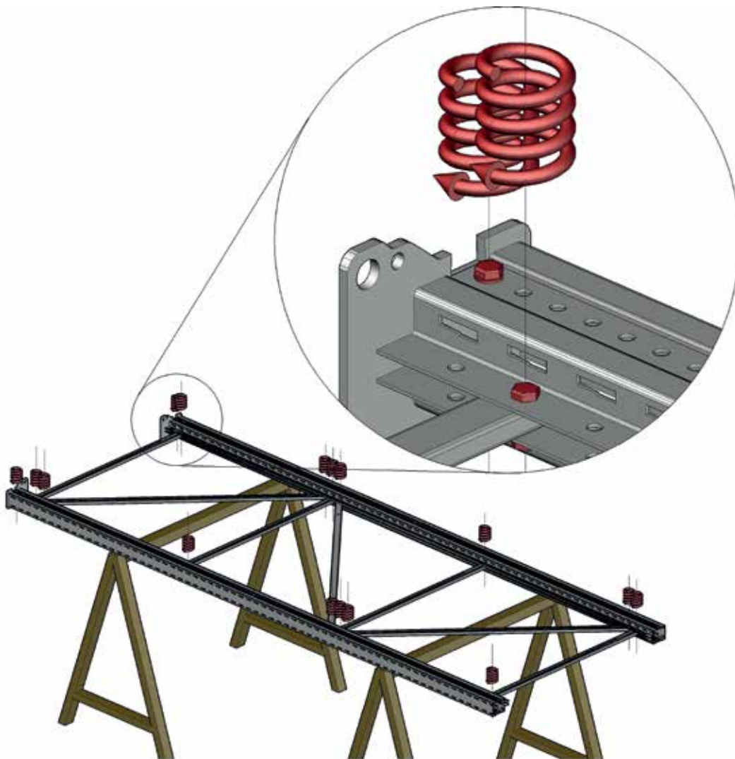
Abb. 61 Montage aller Füllstäbe – Schrauben festziehen
