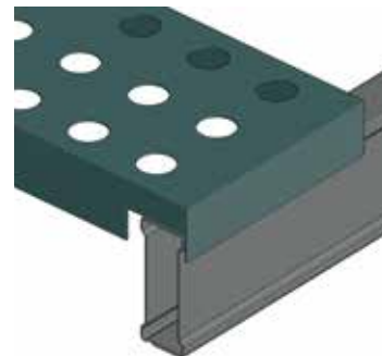
Abb. 37 ITD-Traverse mit aufgelegtem Boden gelocht
