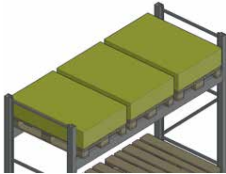
Abb. 78 Gleichmäßig über dem gesamten Traversenpaar verteilte Last
