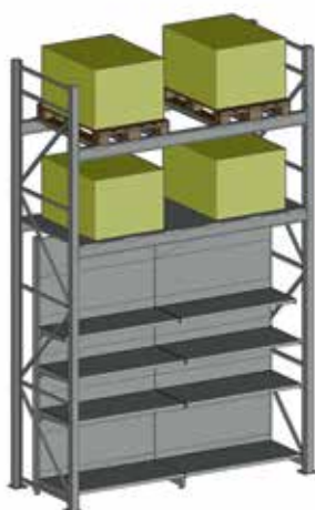
Abb. 3 Regal mit SB-Integrierung lichte Feldweite max. 2636 mm
