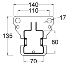
Abb. 17 Standard-Fußplatten der Stützenprofile (alle Maße in mm)
