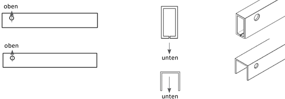
Abb. 52 Montage der Füllstäbe
